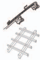
Pose au crochet sur liteaux.
